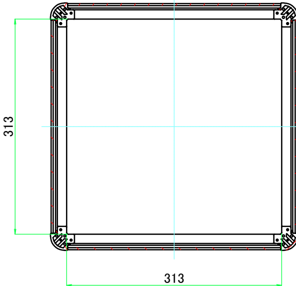
C-C ( 1 : 5.5 )
